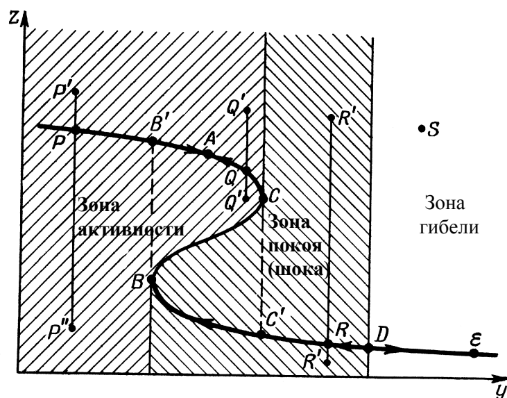
Рис. 7. Фазовый портрет адаптивной системы.
