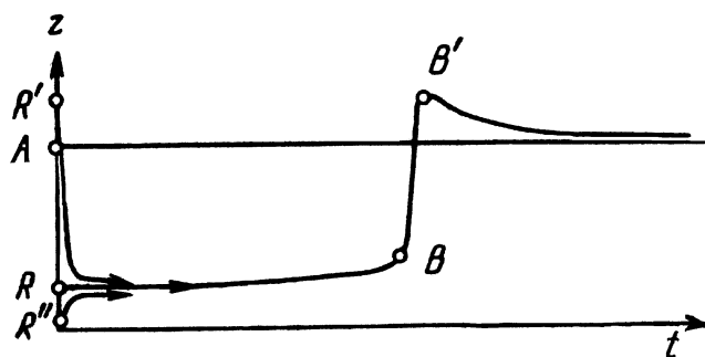
Рис. 10. Лаг-фаза RB и эволюция вдоль линии B'A .
