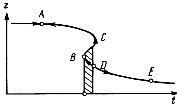
Рис. 12. Устойчивая, но малоадаптивная система.
