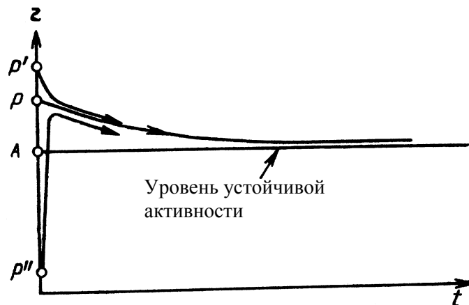
Рис. 8. Сохранение активности и выход на устойчивый режим. Воздействия P, P', P'' .
