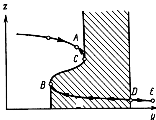
Рис. 13. Адаптивная система с малым запасом устойчивости.
