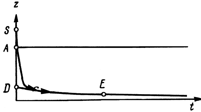
Рис. 11. Необратимые изменения в результате воздействия S . Гибель системы.
