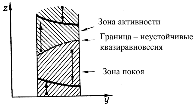
Рис. 5. Состояние неустойчивого квазиравновесия, отделяющее зону активности от зоны покоя.
