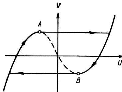
Рис. 1. «Разрывная трактовка» релаксационных колебаний. Пунктиром выделен участок неустойчивости на кривой квазиравновесия. A и B – точки срыва.
