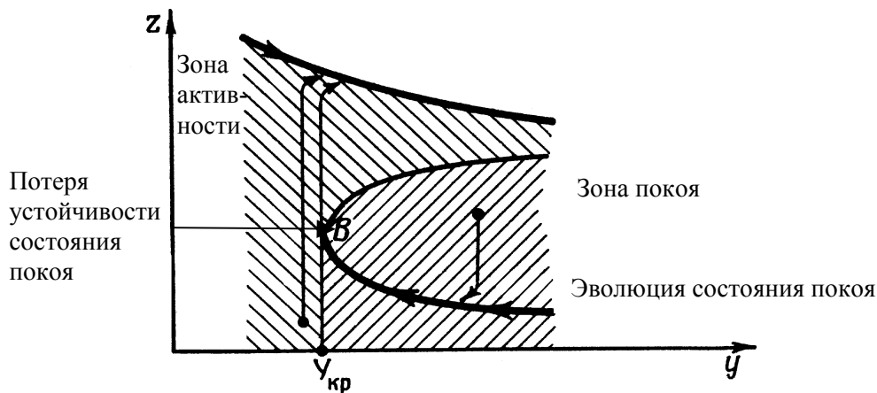
Рис. 6. «Спонтанное» возобновление активности.
