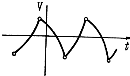
Рис. 3. Изломы в экспериментальной кривой, «выдающие» существование быстрой стадии.
