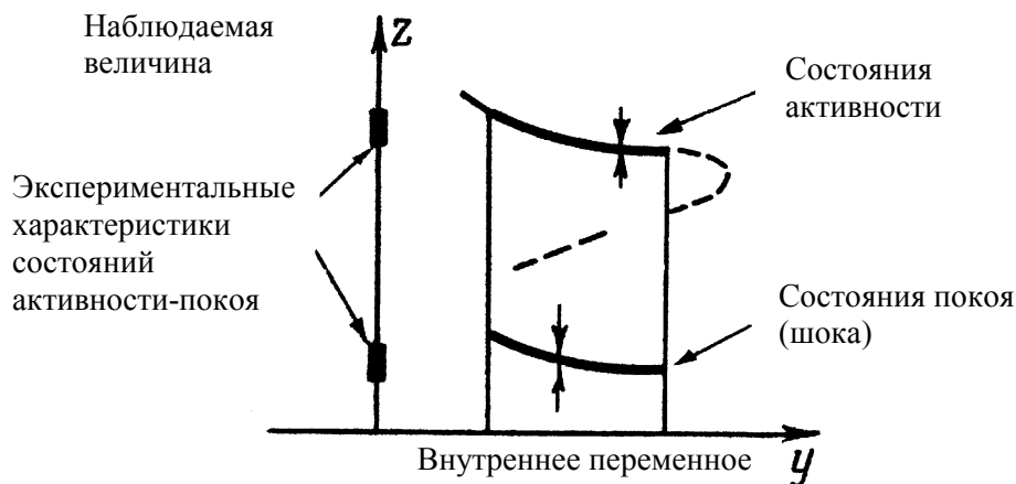
Рис. 4. Две ветви кривой квазиравновесия.
