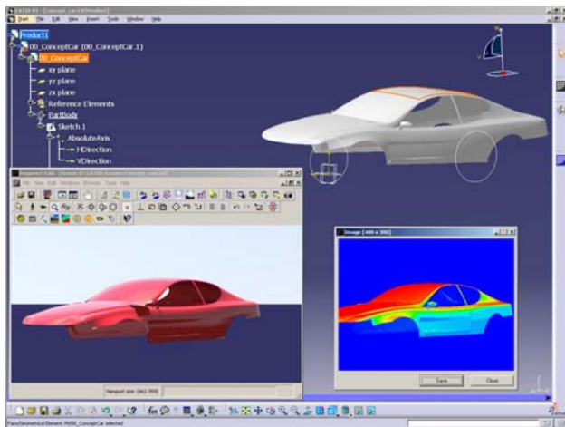
Рис. 2. Результаты интеграции системы моделирования освещенности Inspire2 и системы CATIA.
