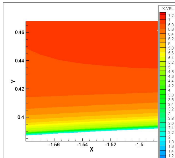
Рис.2. Распределение скорости в пограничном слое.
