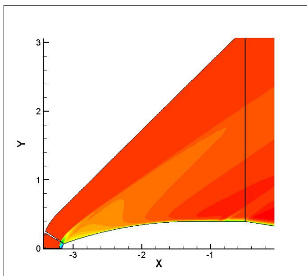
Рис.1. Распределение скорости при обтекании тела вращения.
