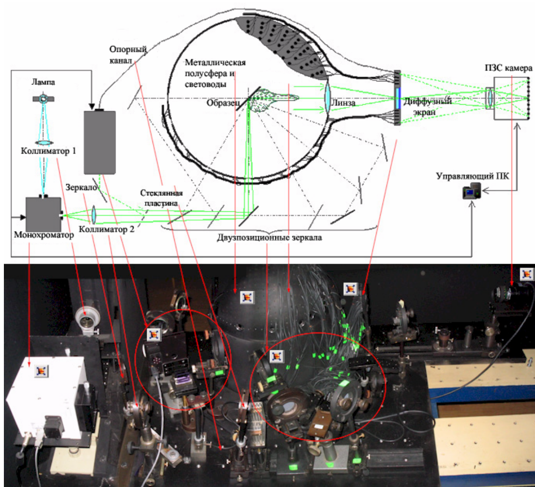
Рис. 5. Схема и общий вид измерительной установки.
