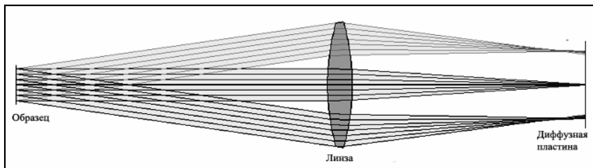
Рис. 8. Преобразование углового распределения в пространственное.
