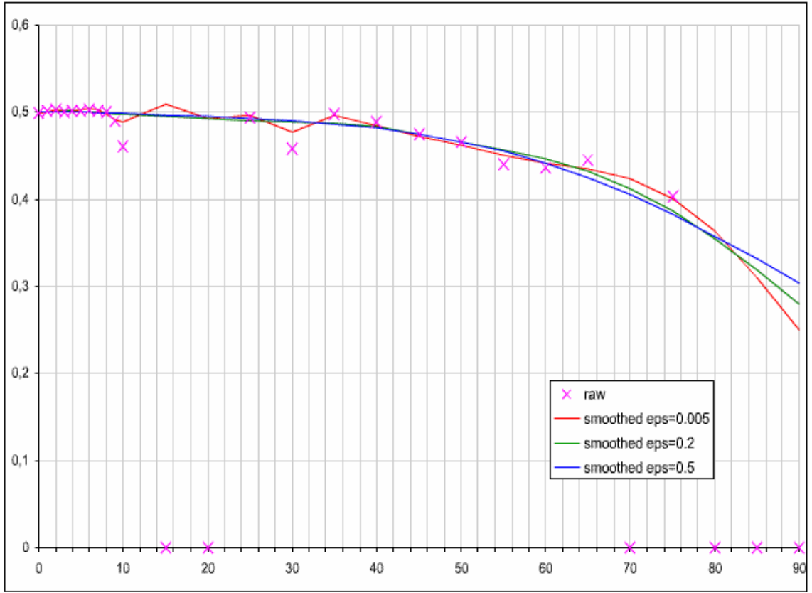
Рис. 11. Аппроксимации первичных данных BDF при различных значениях параметра гладкости \varepsilon .
