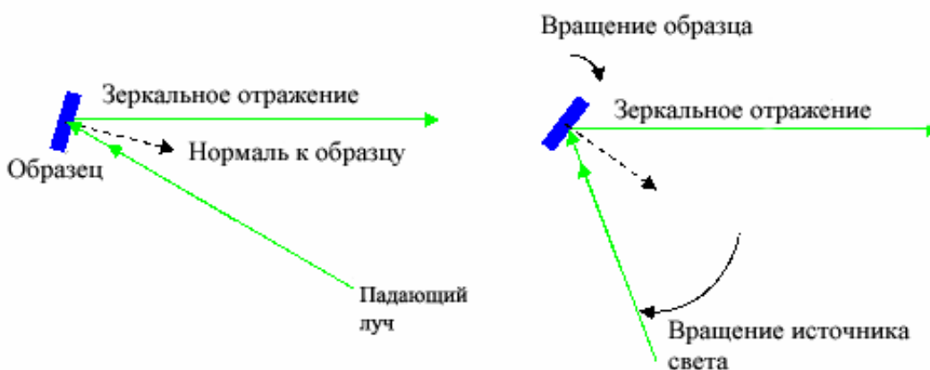
Рис. 7. Изменение направления падающего луча с одновременным вращением образца обеспечивает неизменность направления зеркального отражения.
