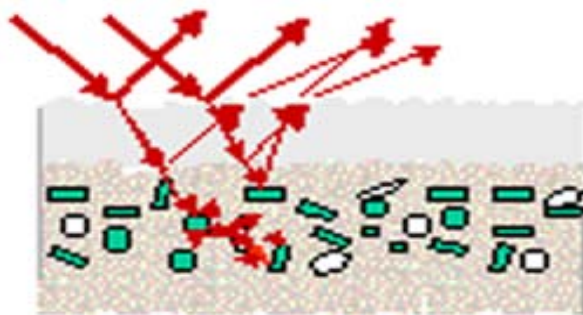
Рис. 3. Объемное рассеяние света в многослойном лакокрасочном покрытии.
