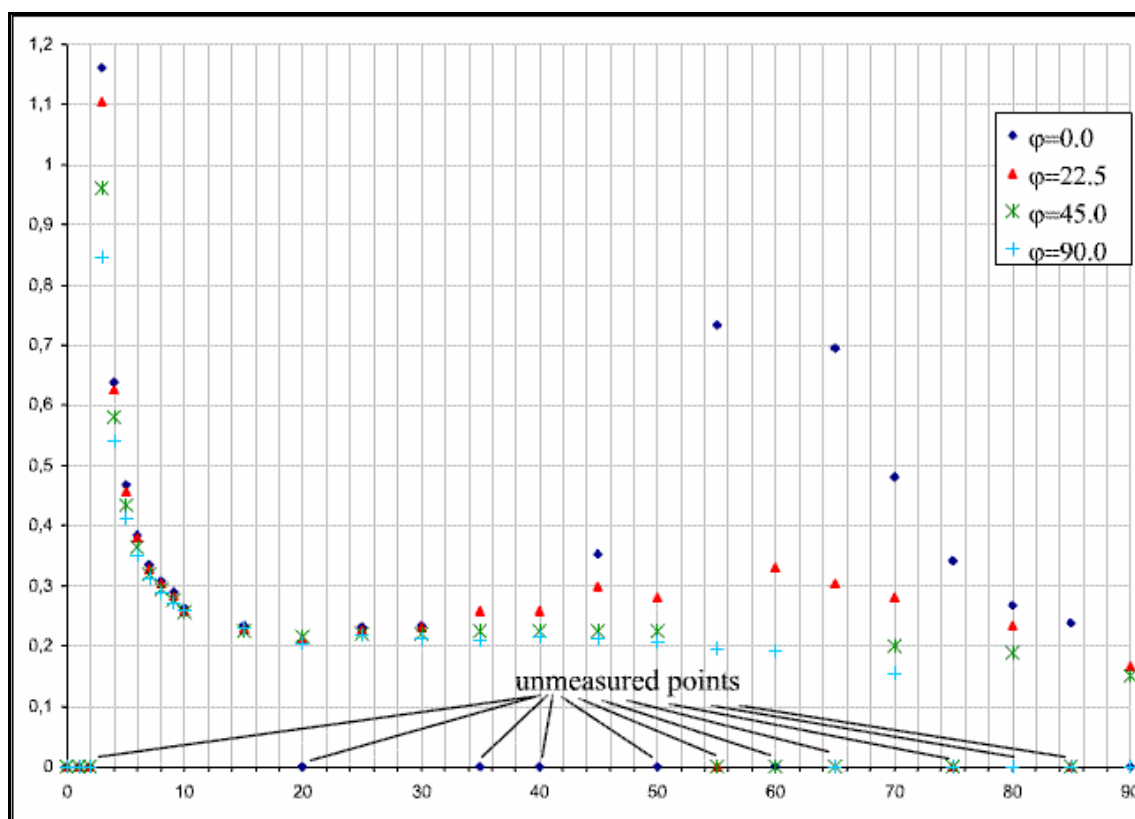
Рис. 10. Пример первичных данных ДФО для \varphi=0^\circ, 22.5^\circ, 45^\circ, 90^\circ .
