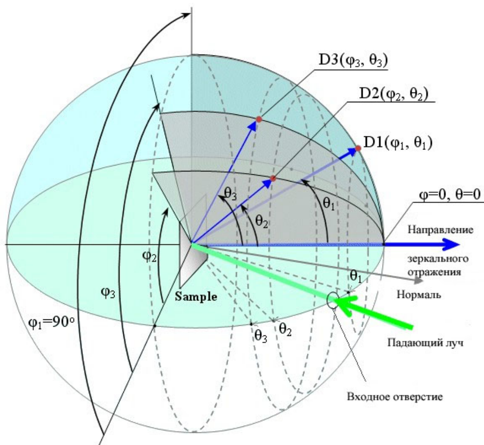
Рис. 6. Сферическая система координат для направлений отраженного света. Направление отраженного света D1 имеет координаты (\varphi_1, \theta_1) , направление D2 - (\varphi_2, \theta_2) и т.д.
