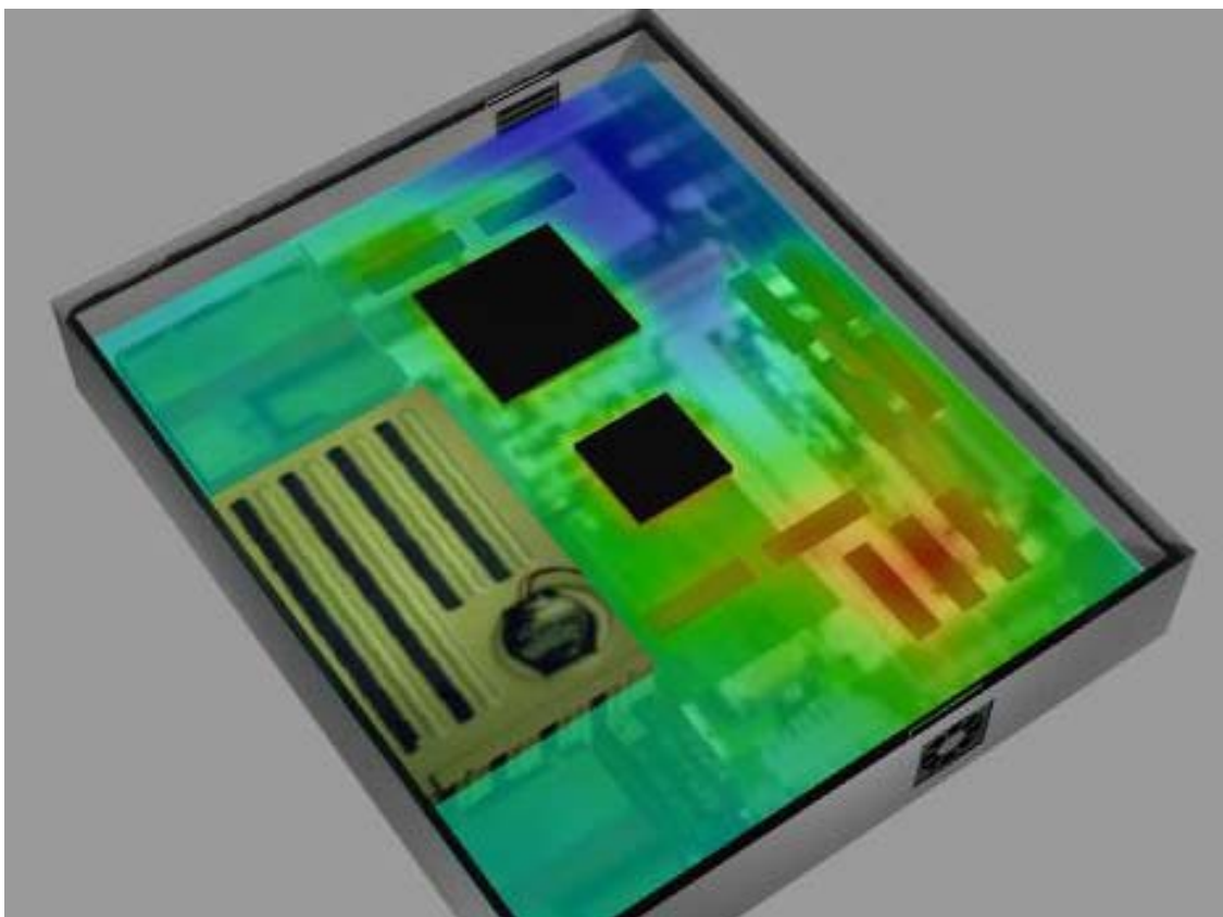
Рис. 4. Распределение температуры в корпусе портативного компьютера
