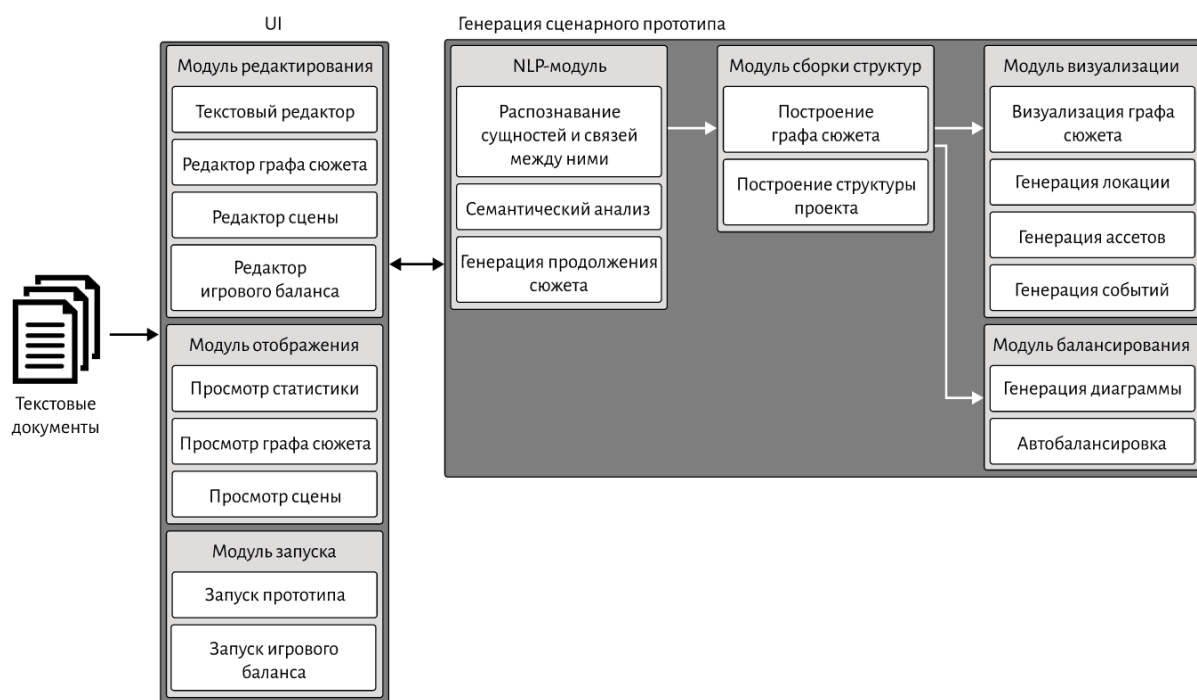
Рис. 9. Структура инструмента генерации сценарного прототипа
