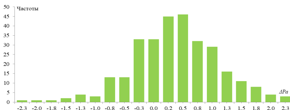
Рис. 5. Гистограмма максимумов для \Delta Pa среднегодового климатического хода
