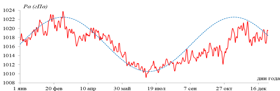
Рис. 3. Поведение среднегодового максимума давления - красная линия; аппроксимация - синий пунктир
