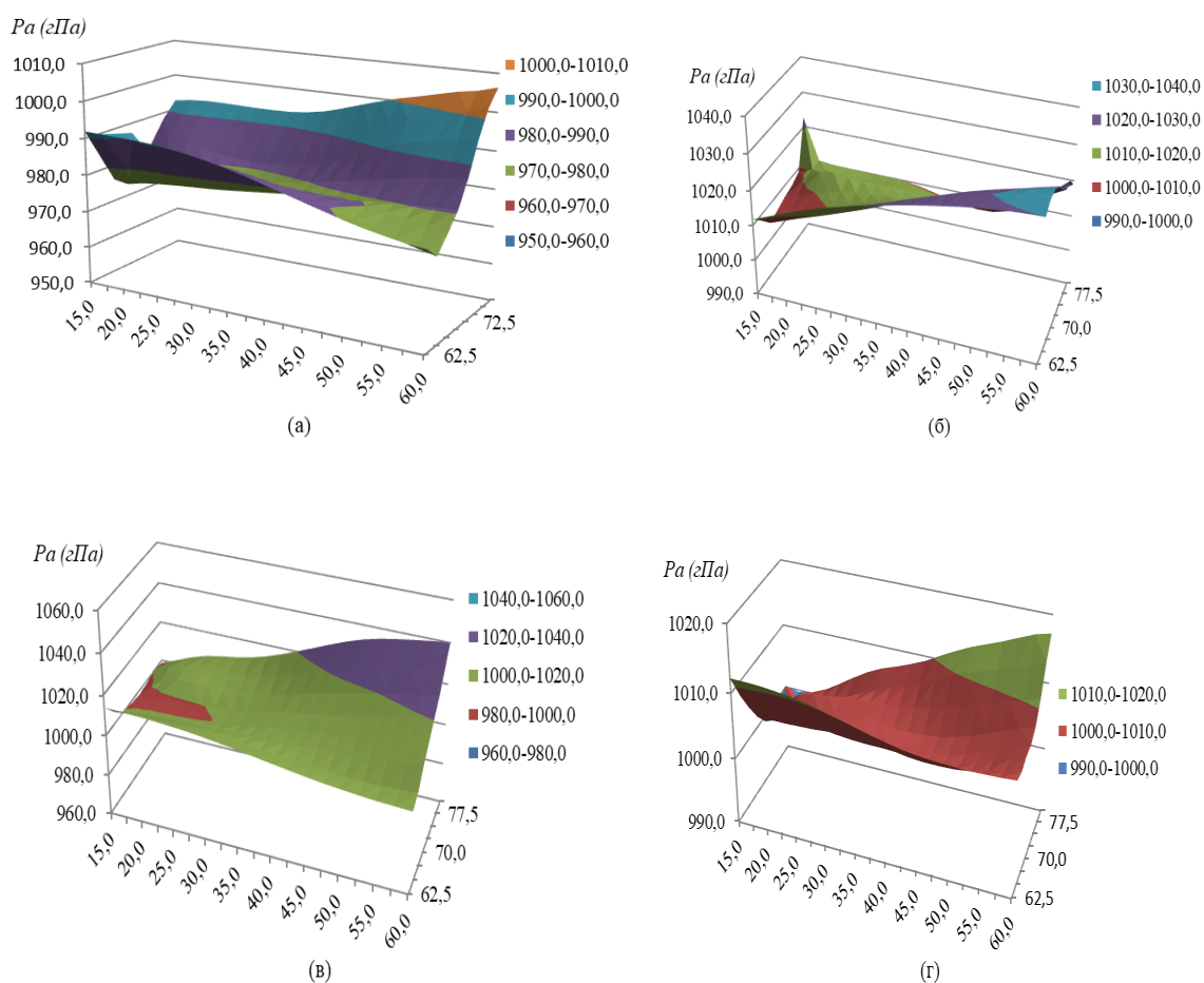
Рис. 2. Поля давления (наблюдения) в Арктической зоне РФ на 1 января: а) 1948 год; б) 1967 год; в) 1987 год; г) 2007 год
