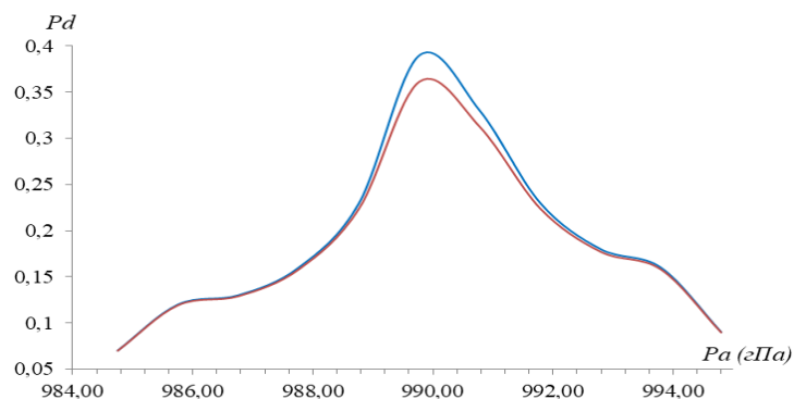
Рис. 9. Аппроксимация случайного остатка минимумов (синяя линия) распределением Максвелла (красная линия)
