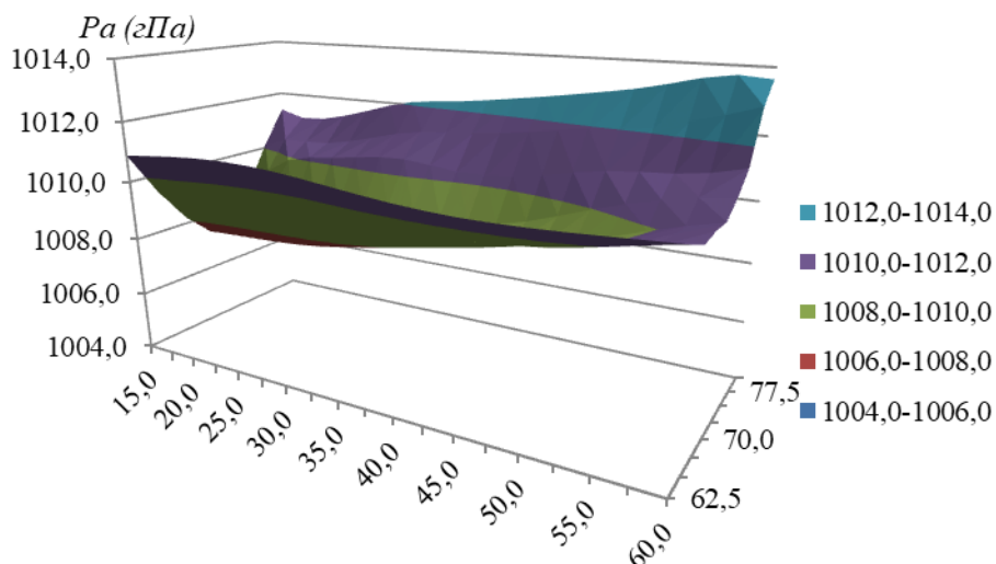
Рис. 2. Поле средних значений давления за 60 лет (01.01.1948 – 31.12.2007) в Арктической зоне РФ
