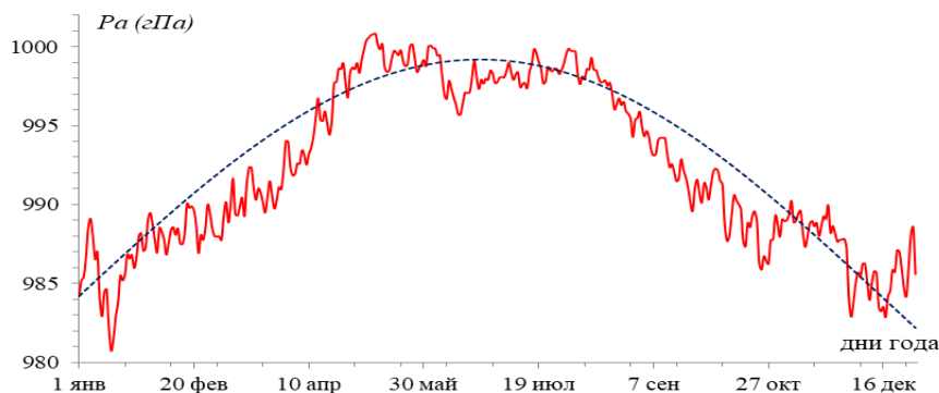
Рис. 7. Кривая средних ежедневных минимумов (красная линия) и аппроксимирующая кривая (синий пунктир)
