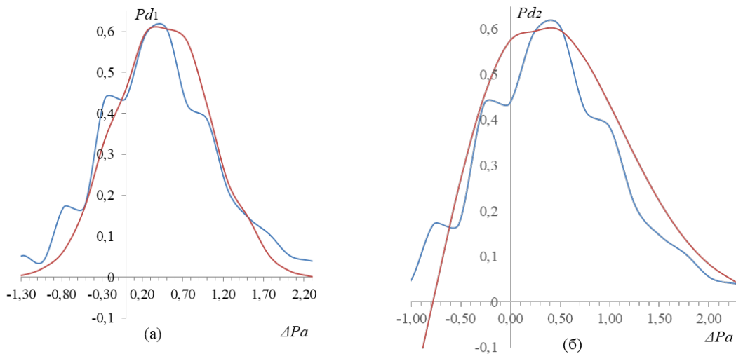
Рис. 6. Аппроксимация случайного остатка максимумов (синяя кривая): распределением: а) Гаусса (красная кривая); б) Максвелла (красная кривая)
