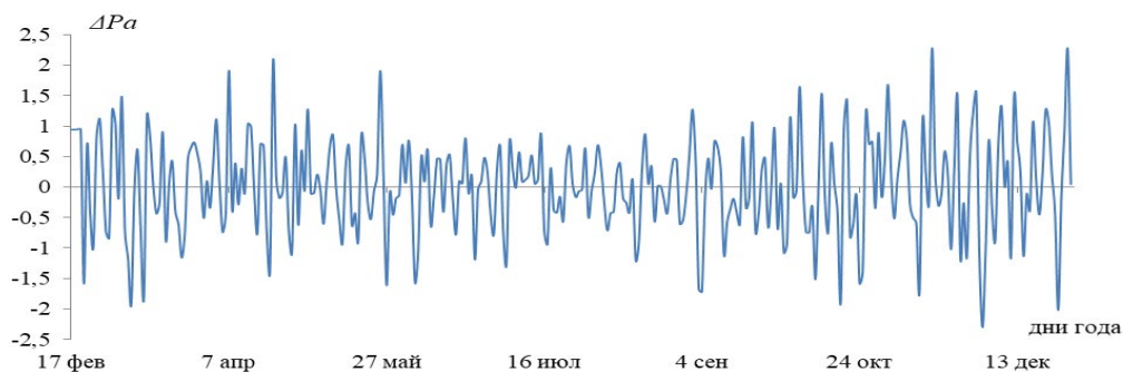
Рис. 4. Разность между наблюдаемой и аппроксимирующей кривой для среднегодового максимума давления
